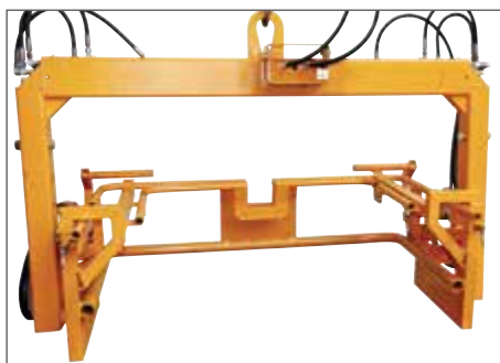
Palonnier hydraulique avec cadre complémentaire pour bac 200 litres
